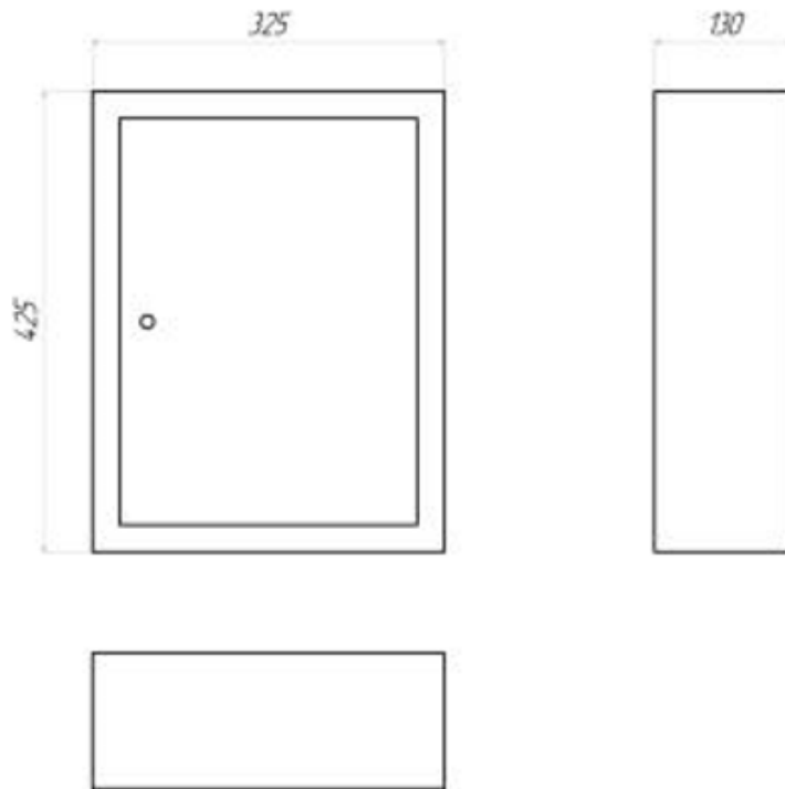
Рис. 1 Габаритні розміри.
