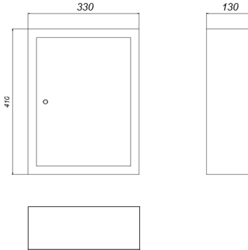
Рис. 1 Габаритні розміри.
