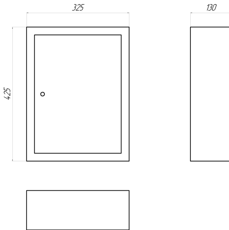
Рис. 1 Габаритные размеры.
